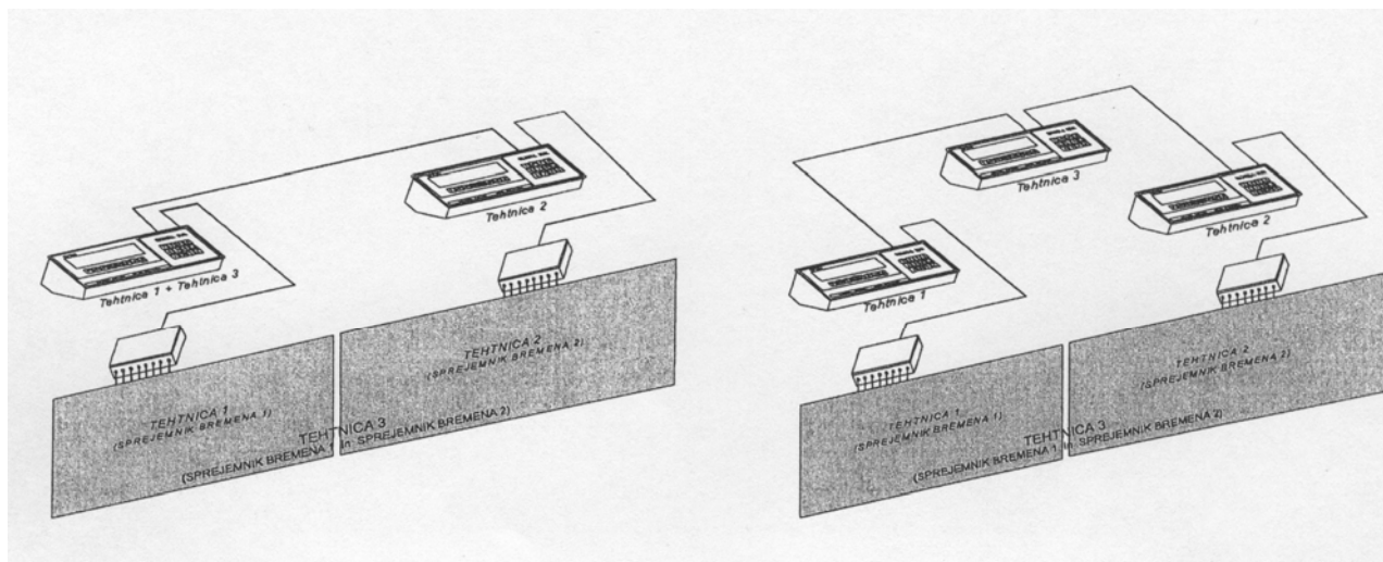
Slika 2: Shema povezave dveh tehtnic v sistem in shema povezave dveh tehtnic in dodatne elektronske naprave v sistem.
